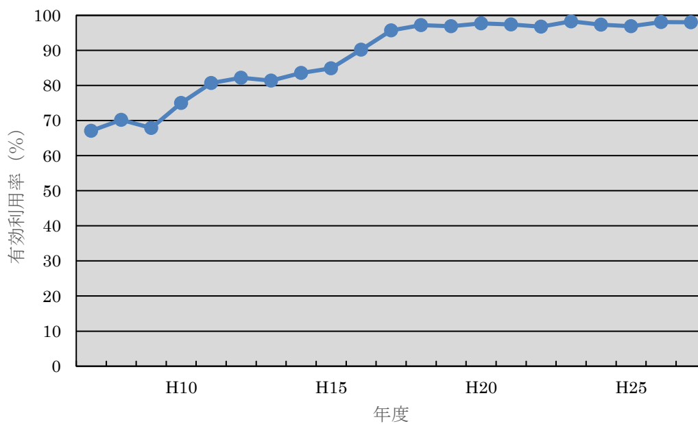
図4 石炭灰の有効利用率
