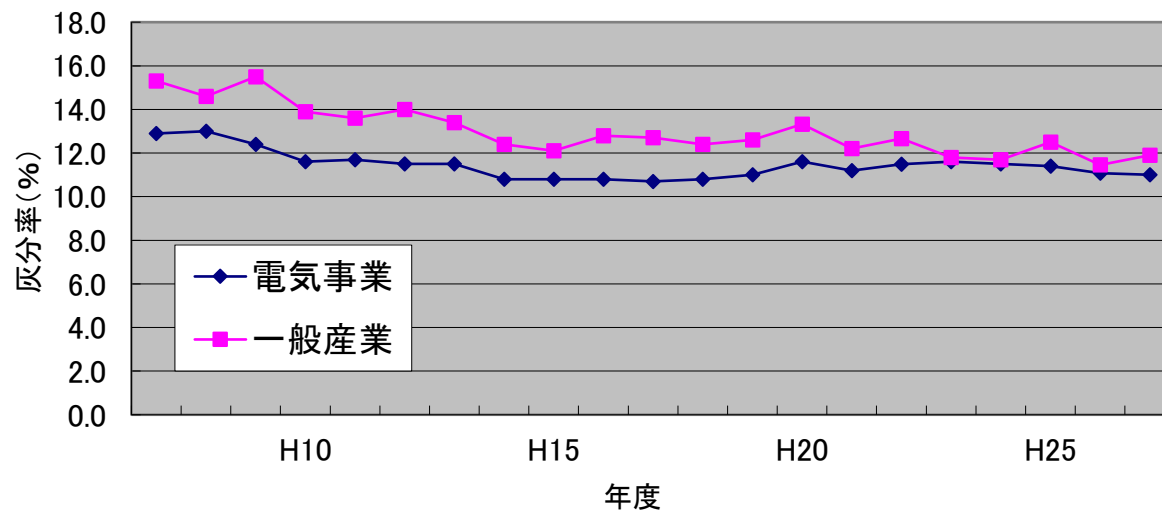
図2 石炭中の灰分（平均値）の推移
